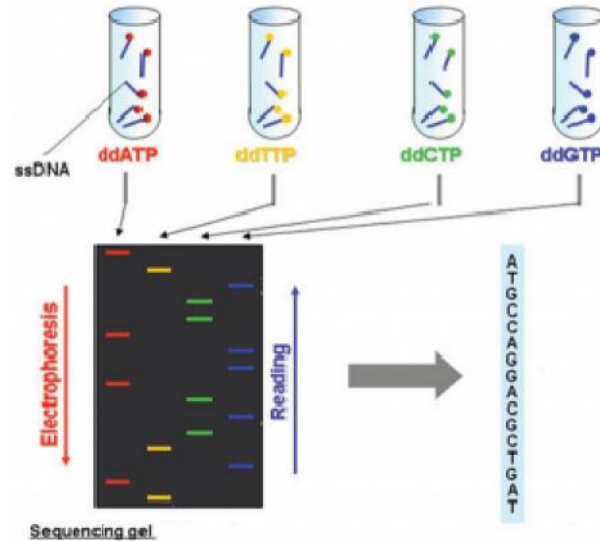
شکل 2- نحوه خواندن نوکلئوتیدها از روی ژل الکتروفورز
