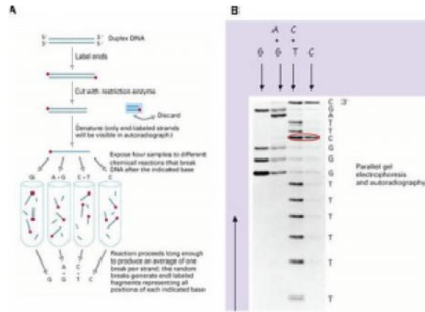
شکل 3- تعیین توالی به روش ماکسام - گیلبرت
